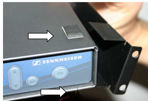
A- Dévissez la plaque de masquage. B- Collez les pieds adhésifs en quatre emplacements.
