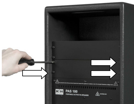
A- Dévissez la plaque de masquage. B- Collez les pieds adhésifs en quatre emplacements.
