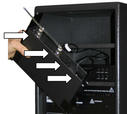
(D) Befestigen Sie die Audio-, Strom- und Antennenstecker am Empfänger
