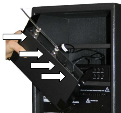
D- Effectuez les branchements : alimentation, 2 antennes, audio.
